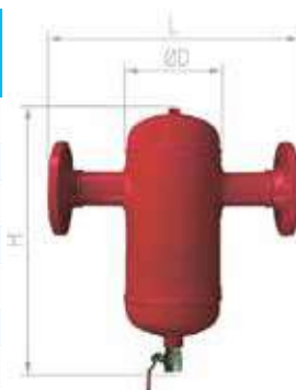
Conexión EMBRIADAS
